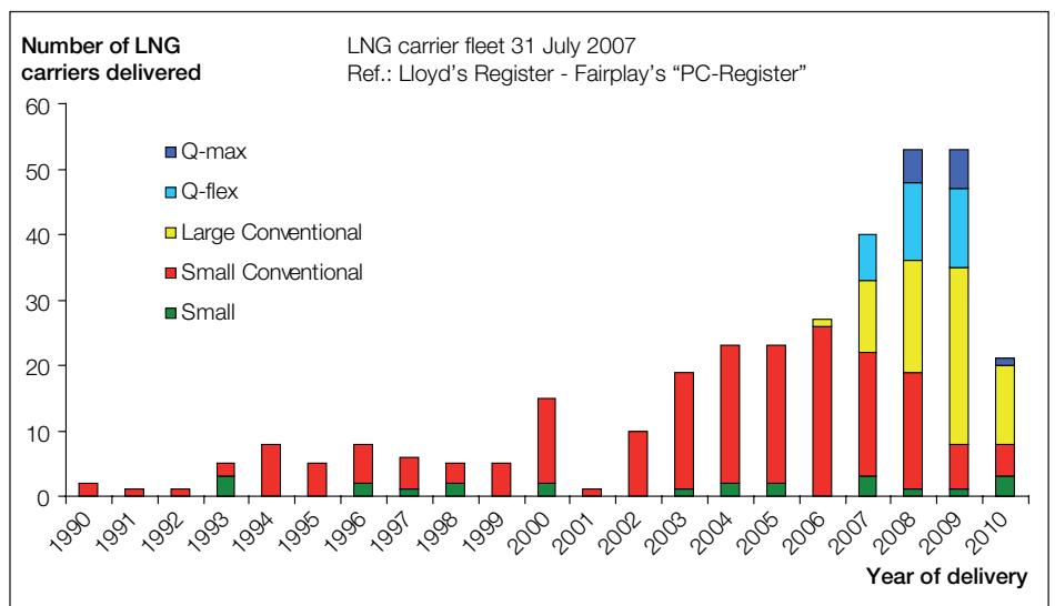
Fig. 4c: Year of delivery of LNG carriers
