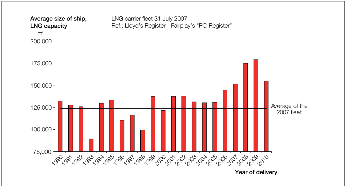
Fig. 4d: Average size of LNG carriers delivered
